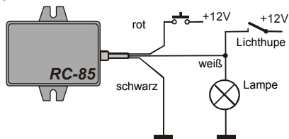
Beispiel einer Verdrahtung in einem Fahrzeug
