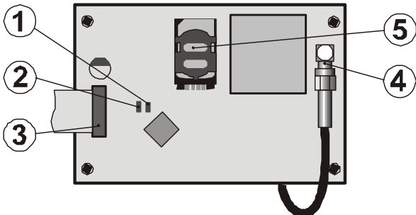
1.LED GSM-Netz 2.LED Foto-Übertragung 3. Anschluss Zentrale 4. Anschluss GSM-Antenne 5. SIM-Karten-Halterung
