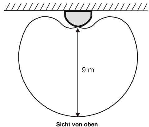
Erfassungsbereich des Glasbruchsensoren
